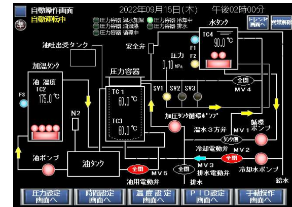
6 冷却中
