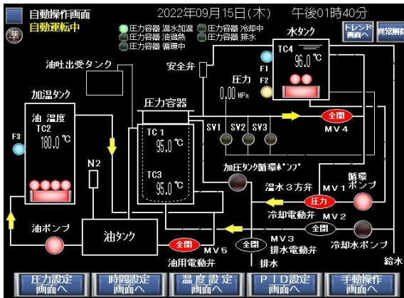
3 温水循環
